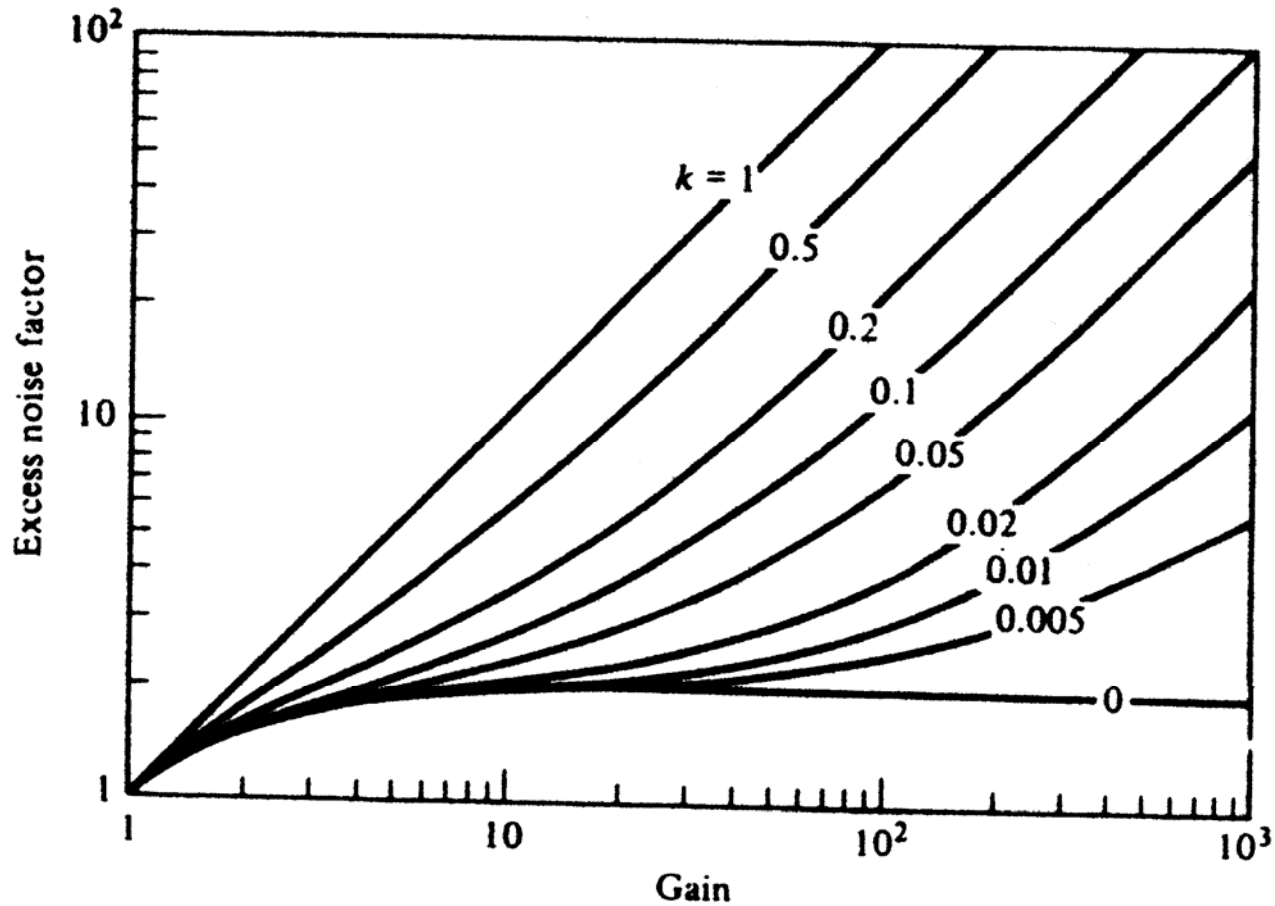
Variasi faktor noise electron excess sbg fungsi dr penguatan elektron utk berbagai harga perbandingan laju ionisasi efektif k_{\text{eff}}
